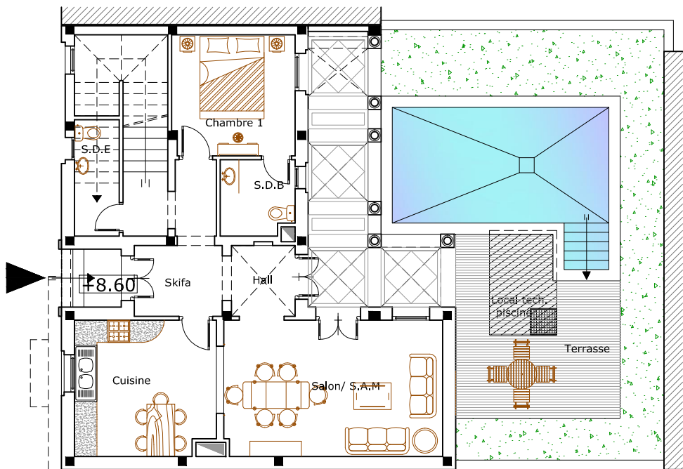
Plan R.D.C
